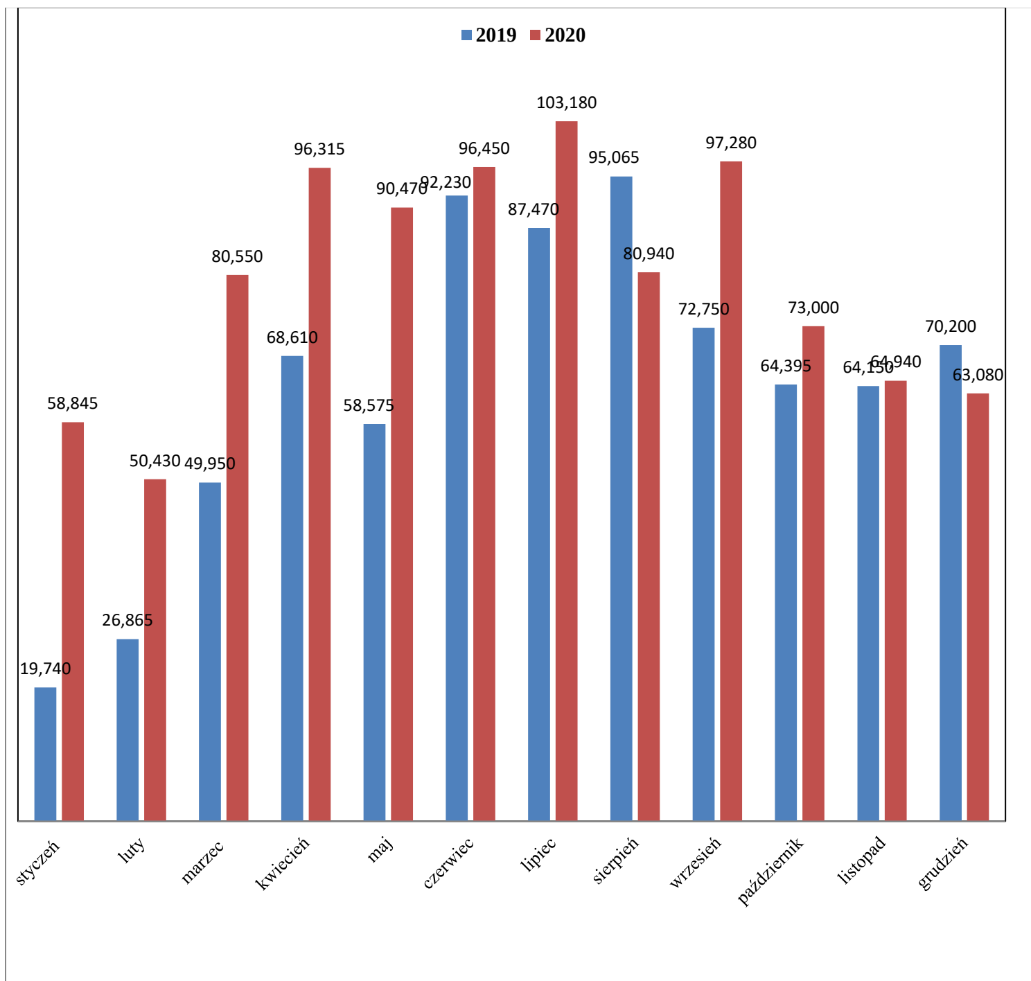
Wykres 1 Porównanie ilości odpadów zebranych z PSZOK-u w 2019 i 2020 roku.
