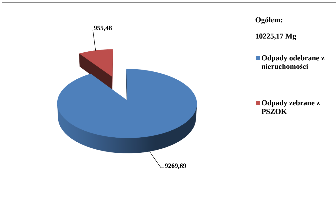
Wykres 5 Ilość odpadów z nieruchomości oraz zebranych z PSZOK
