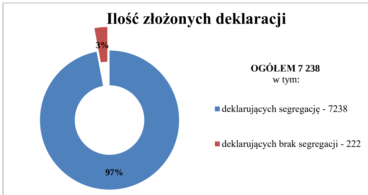
Wykres 2 Ilość złożonych deklaracji o wysokości opłaty za gospodarowanie odpadami komunalnymi - stan na dzień 31 grudnia 2020 r.
