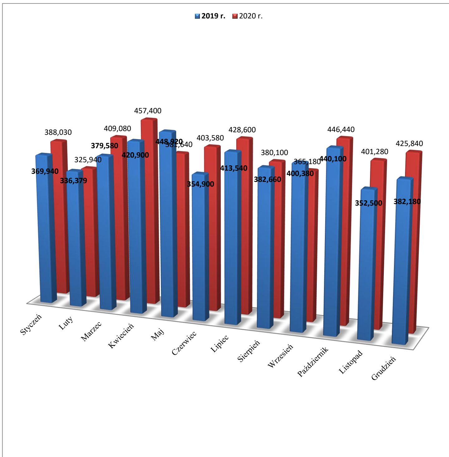
Wykres 4 Ilość odebranych odpadów komunalnych niesegregowanych w 2019 oraz 2020 roku w Mg.
